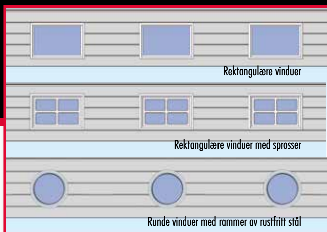
FORSKJELLIGE VINDUSTYPER
